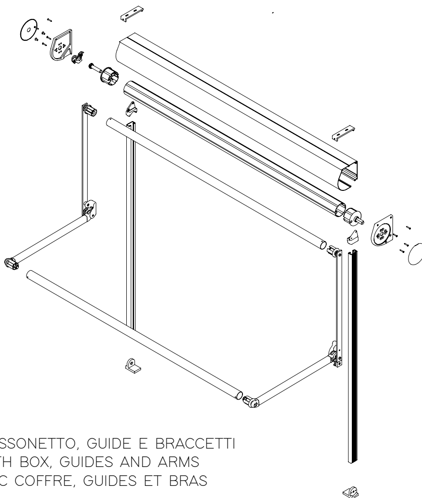
VENEZIA CON CASSONETTO E CAVETTO / ASTA VENEZIA WITH BOX AND CABLE / ROD VENEZIA WITH BOX AND CABLE / TIGE
